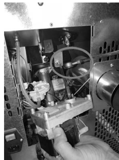
Fig. 72 - Rimozione motoriduttore
