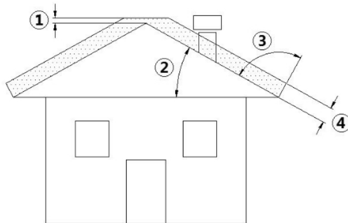
Fig. 3 - Tetto inclinato
