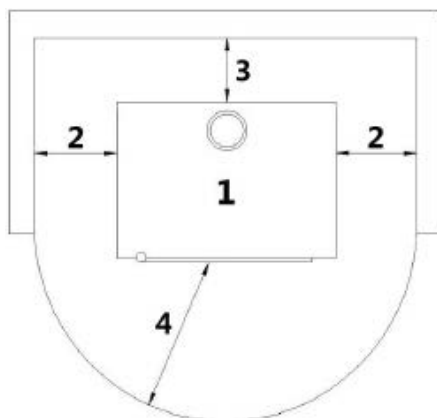
Fig. 23 - Installazione generica
